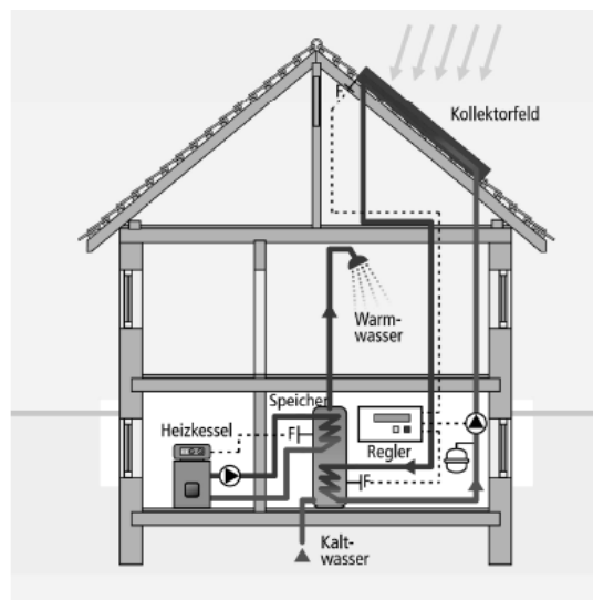
Bild: BFE, Schema Haustechnik mit Solarthermie
